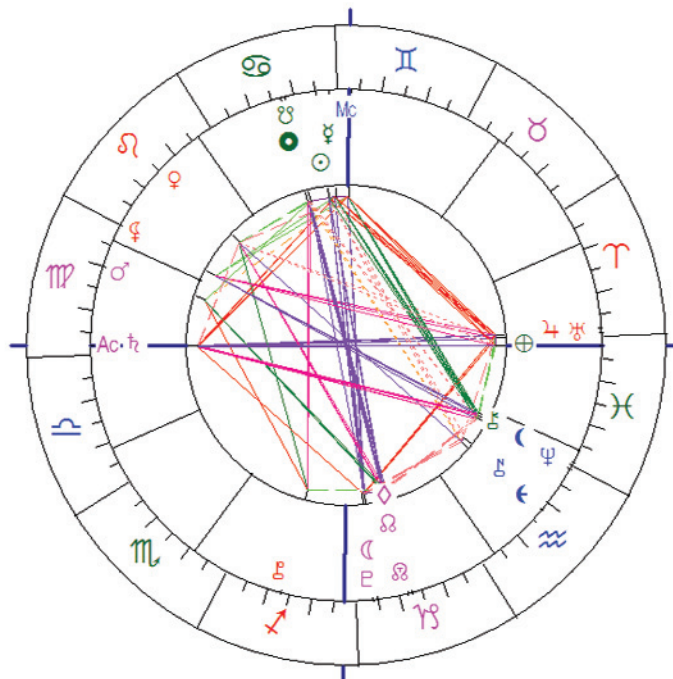
De gedeeltelijke maansverduistering van 26 juni 2010 12:30 MET Greenwich.
